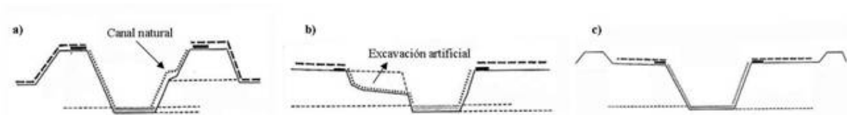
Figura J.2. Ejemplos de las elevaciones artificiales de los márgenes fluviales: a) sobre-elevación de las orillas, b) escalonado artificial, c) elevación de la llanura de inundación.
